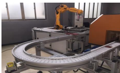
基于机器人的鞋品智能化生产线
